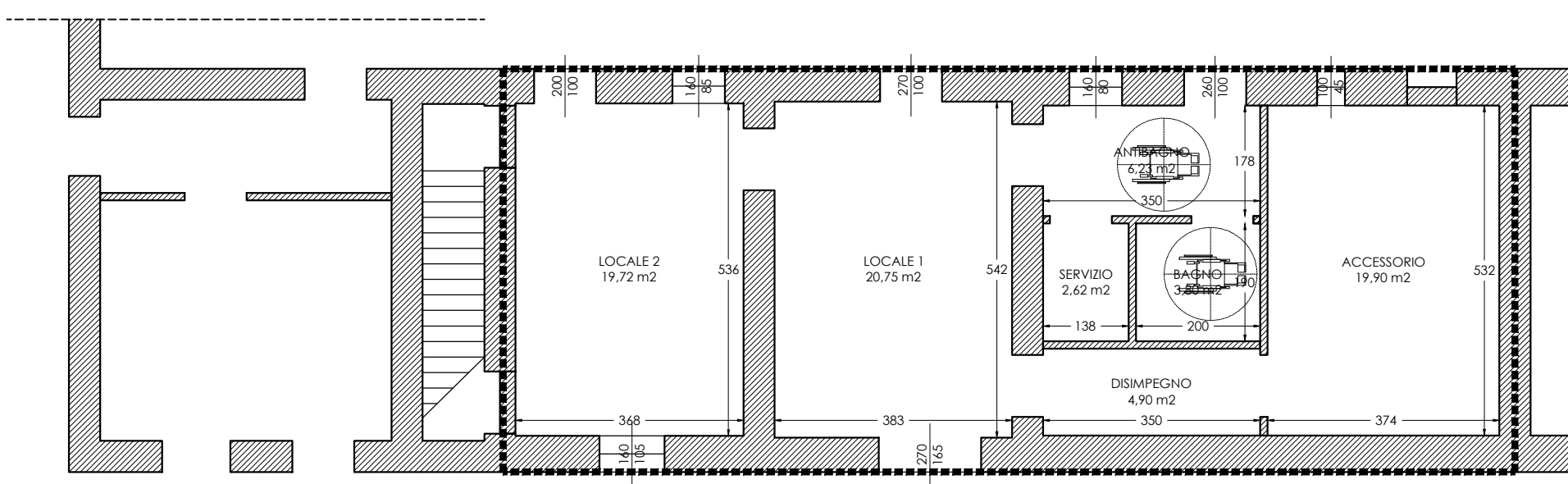
FABBRICATO "CASA VOLPI" - PIANO TERRA 27020 ALAGNA (PV) - CORSO VITTORIO VENETO N. 48 SCALA 1:100
